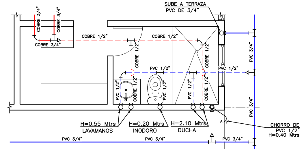
2 DETALLE 1 SANITARIO DORMITORIO 1 ESCALA: 1:50
