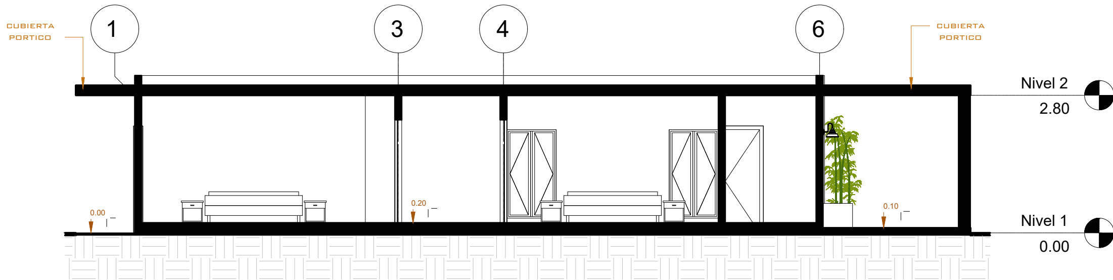
4 SECCIÓN LONGITUDINAL 2 1 : 75
