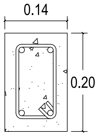
COLUMNA A 4 Ø1/2" + est. Ø1/4" @ 0.15
