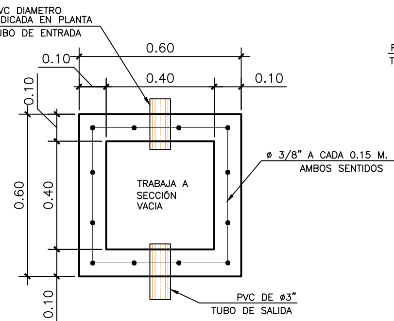
4 PLANTA CAJA DE UNION CU2
