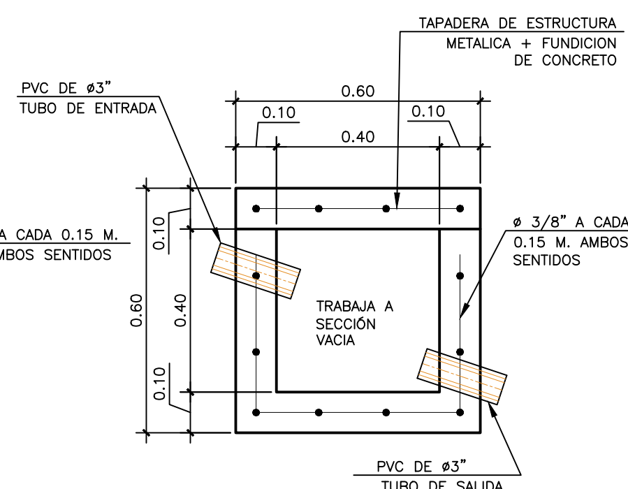
5 ELEVACION CAJA DE UNION CU2 ESCALA: 1:2.5
