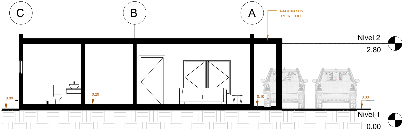
3 SECCIÓN TRANSVERSAL 2 1 : 75
