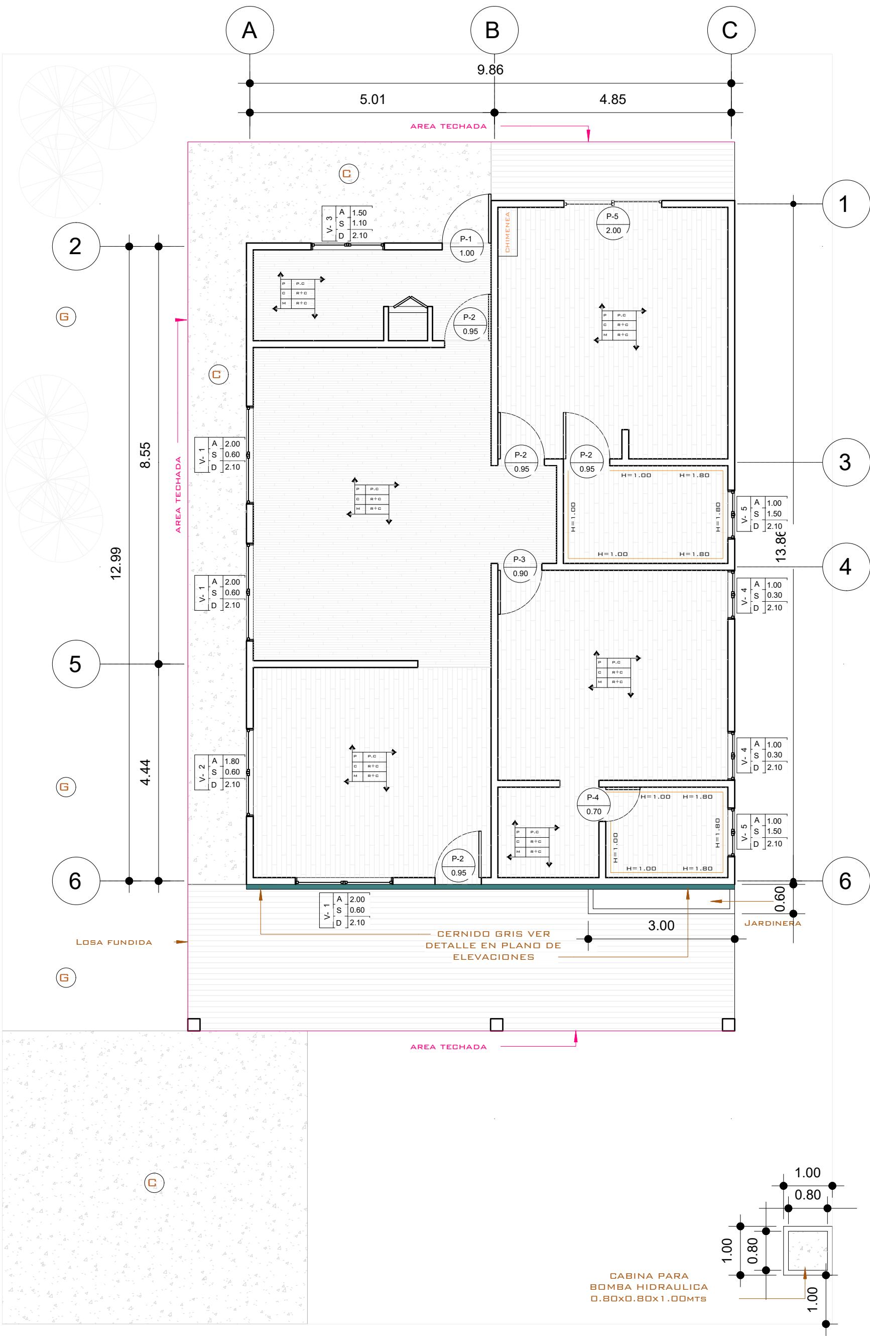
1 PLANTA NIVEL 1 DE ACABADOS ESCALA: 1:100
