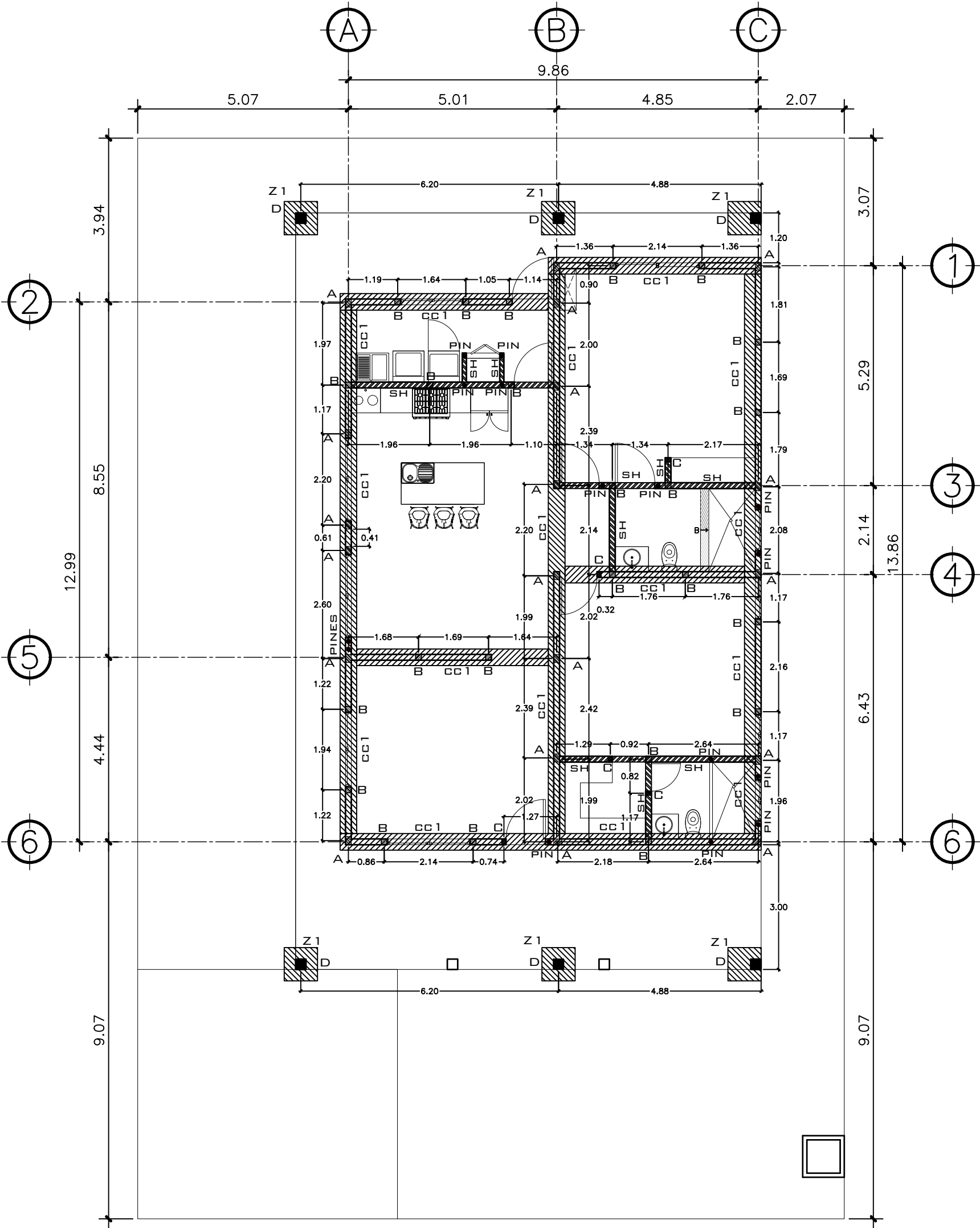
1 PLANTA NIVEL 1 CIMENTACION Y COLUMNAS ESCALA: 1:100
