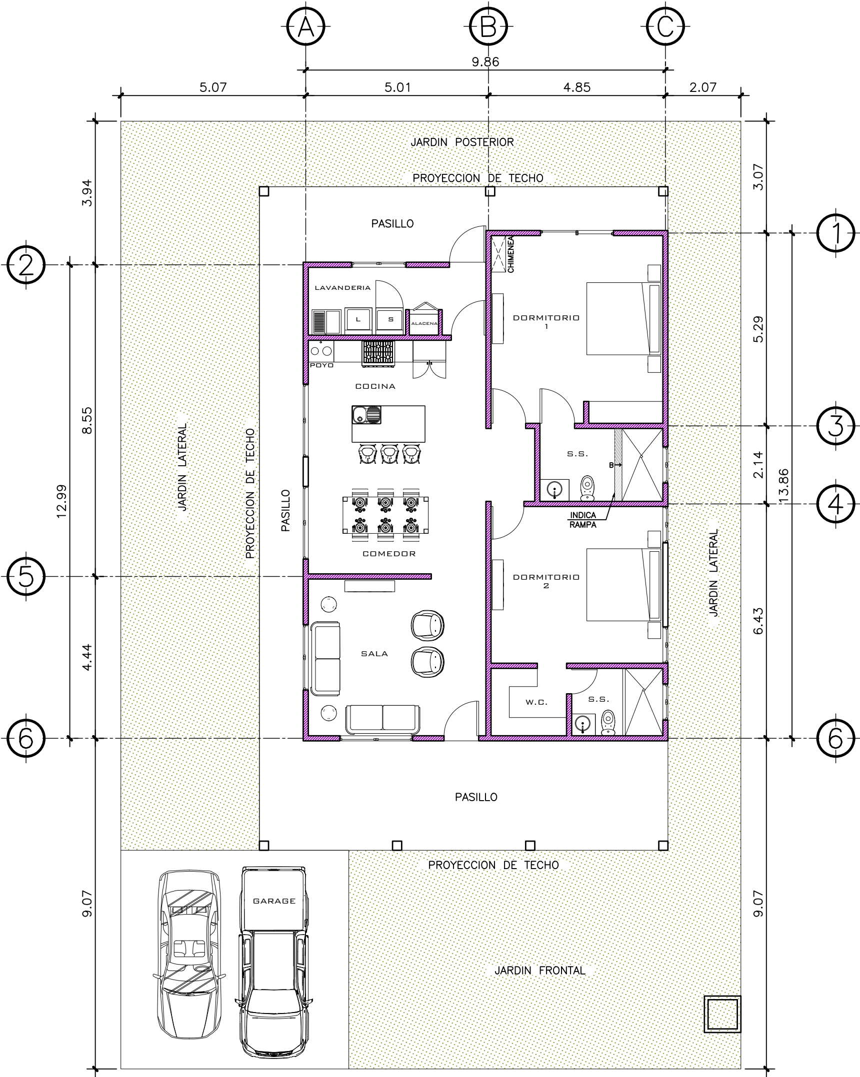
1 PLANTA NIVEL 1 AMOBLADA ESCALA: 1:100
