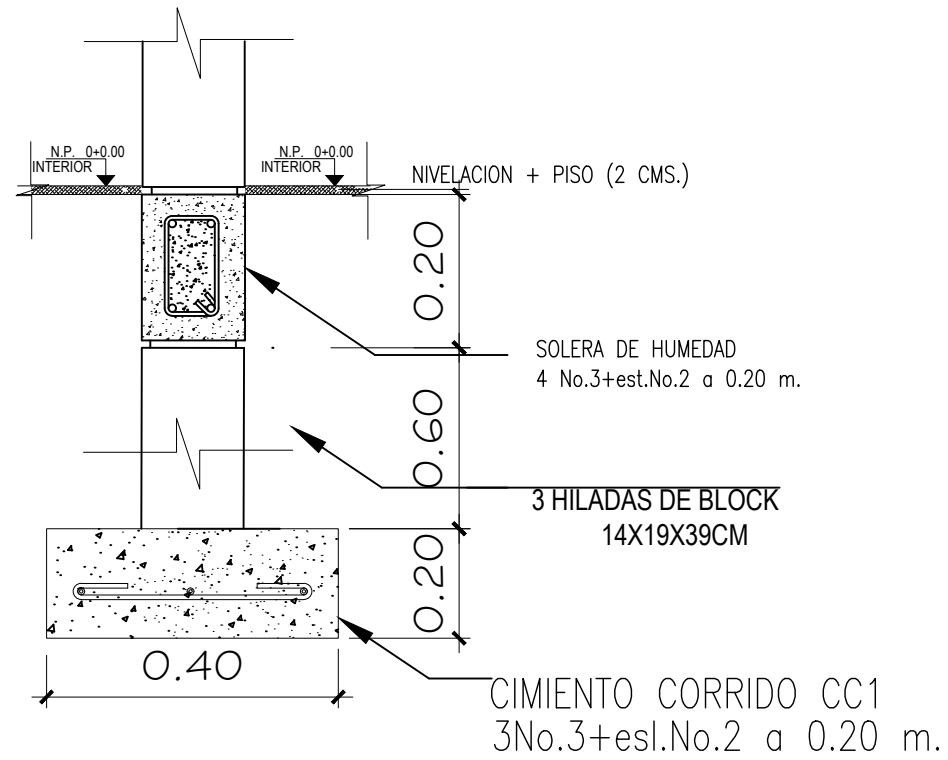
CIMIENTO CORRIDO CC 1
