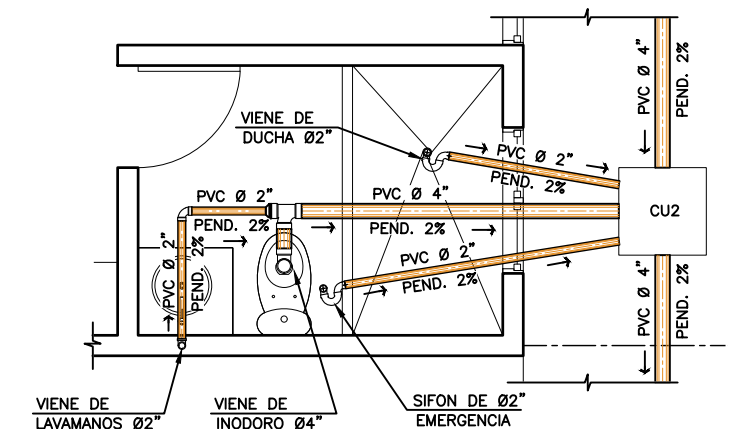
3 DETALLE 2 SANITARIO DORMITORIO 2 ESCALA: 1:50
