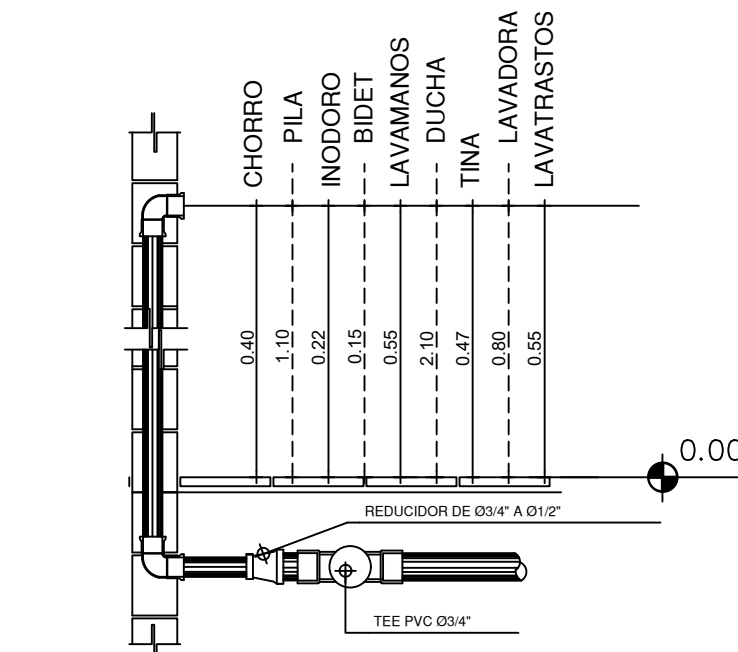
3 DETALLE TIPICO DE ALTURAS ESCALA: 1:75
