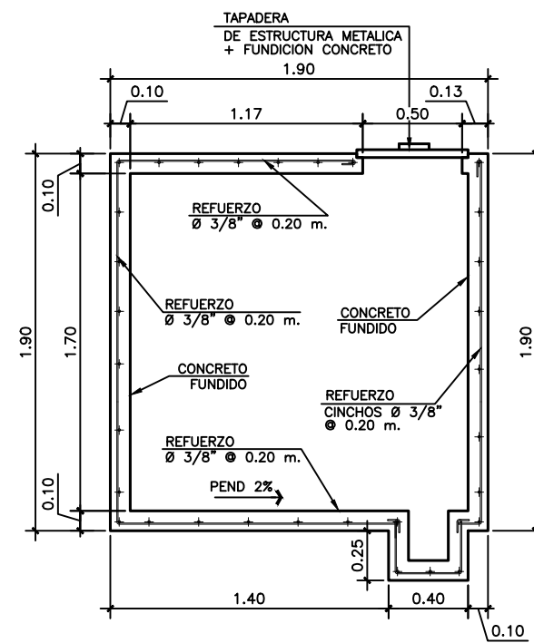
5 SECCION 1 ARMADURA DE CISTERNA + ACOTADA ESCALA: 1:25
