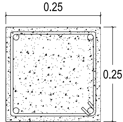
COLUMNA D 4 Ø5/8" + EST. Ø1/4" @ 0.15
