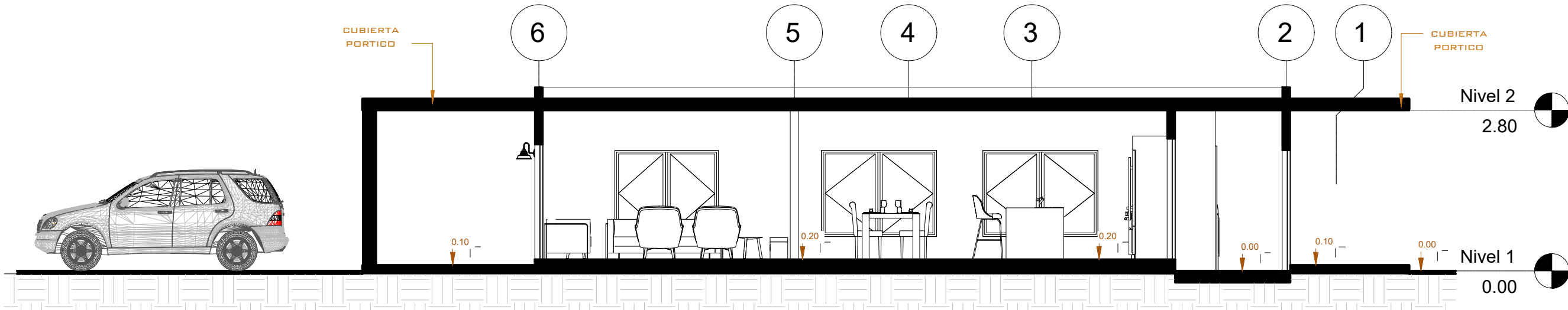
1 SECCIÓN TRANSVERSAL 1 : 75
