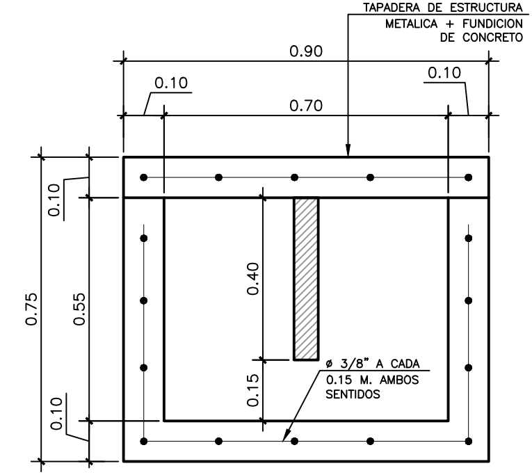
9 ELEVACION CAJA TG ESCALA: 1:2.5
