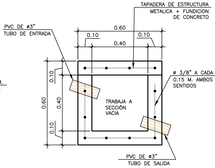
5 ELEVACION CAJA DE UNION CU2
