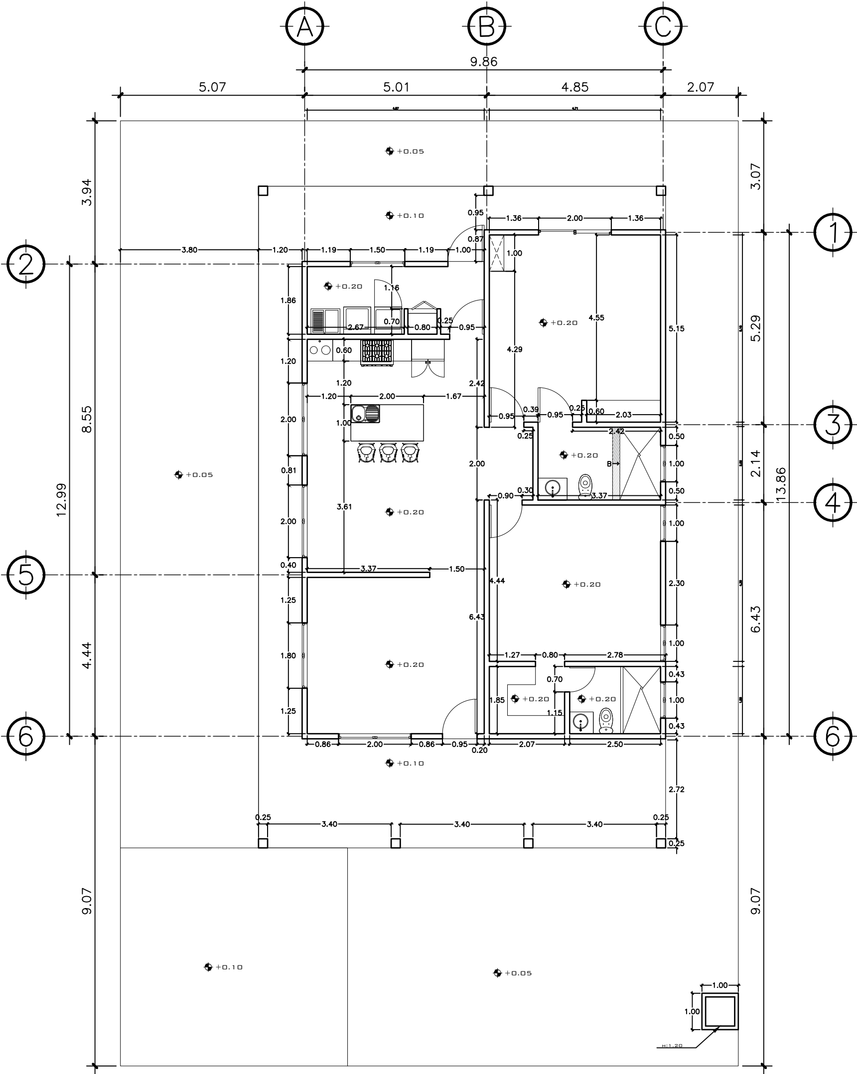
1 PLANTA NIVEL 1 ACOTADA ESCALA: 1:100
