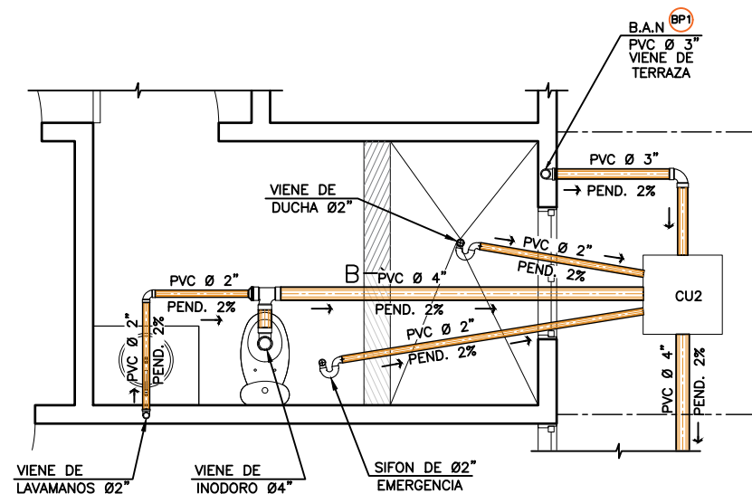
2 DETALLE 1 SANITARIO DORMITORIO 1 ESCALA: 1:50
