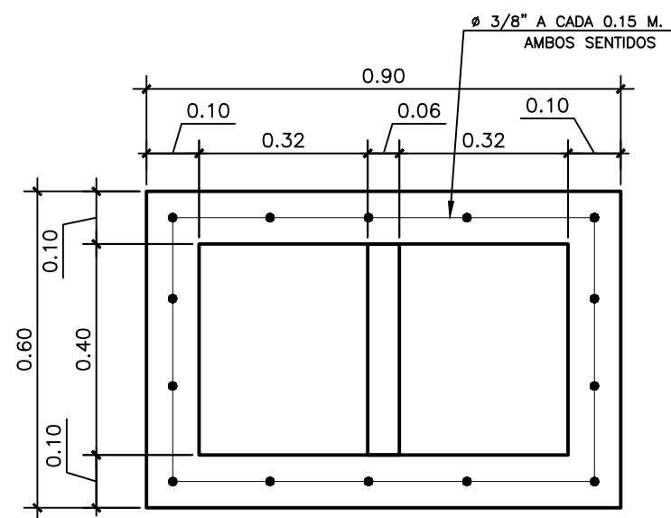
8 PLANTA CAJA TG ESCALA: 1:2.5
