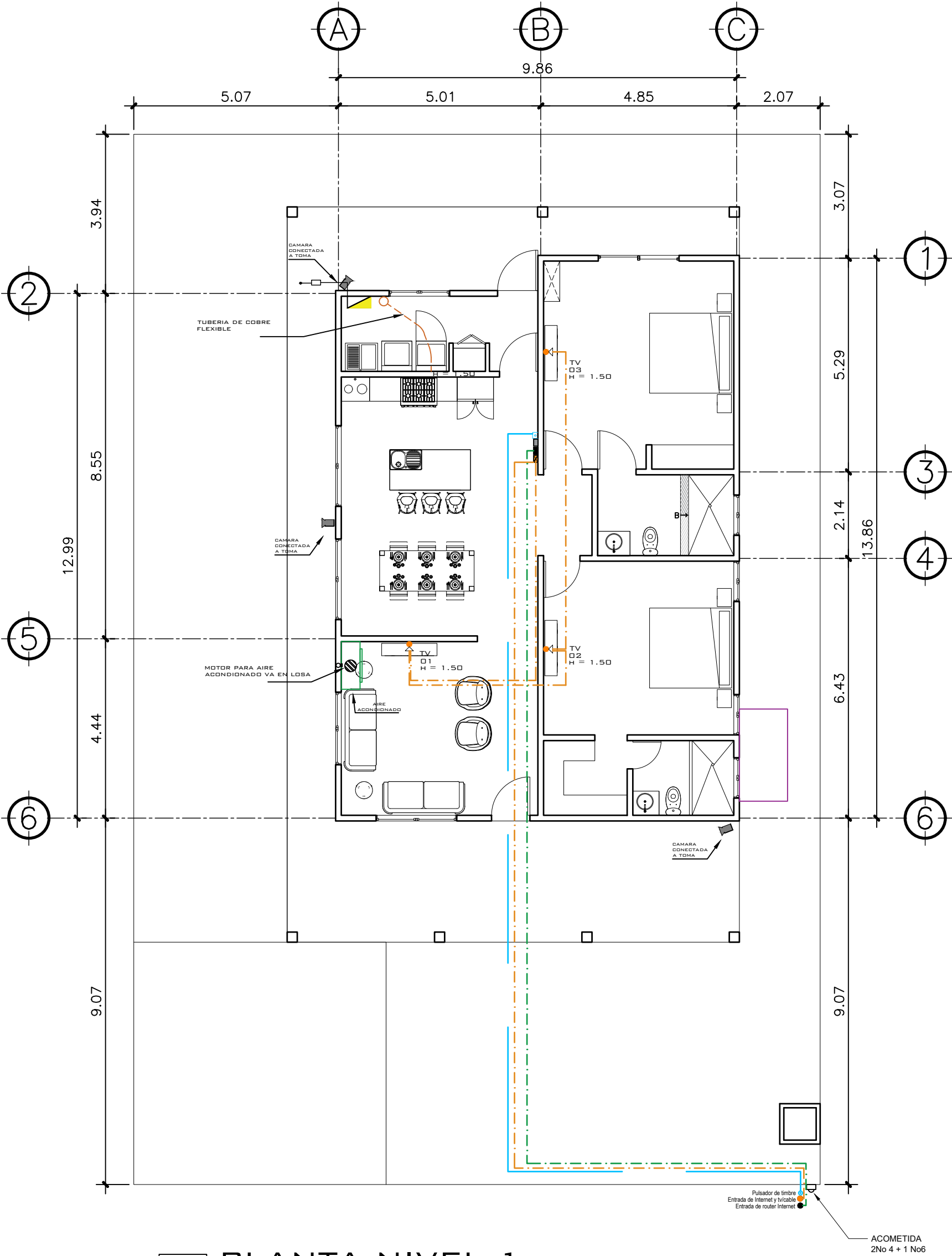
1 PLANTA NIVEL 1 ESPECIALES ESCALA: 1:100
