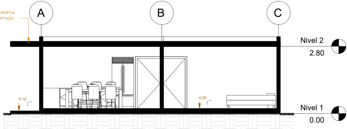
1 SECCIÓN TRANSVERSAL 1 : 75
