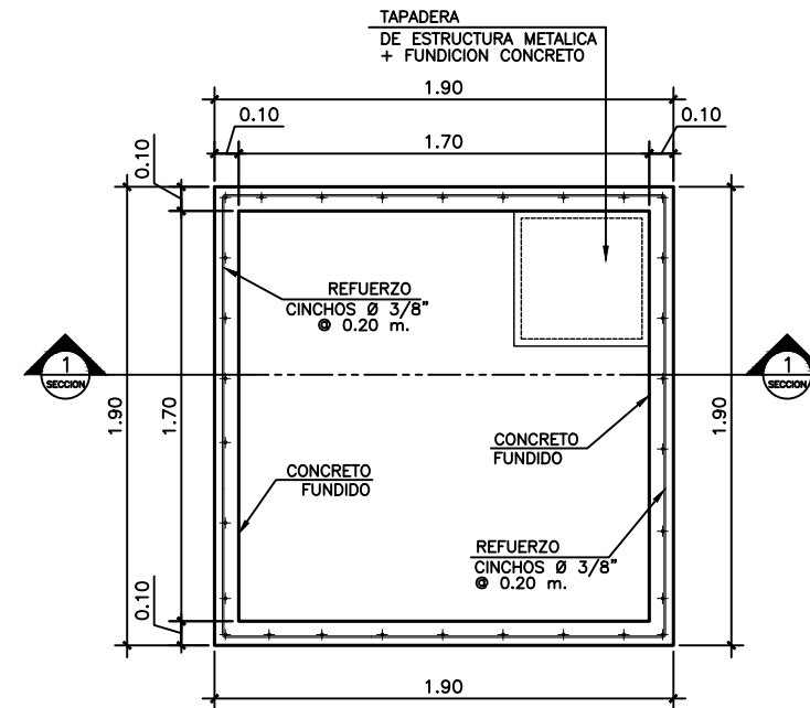
3 DETALLE 2 SANITARIO DORMITORIO 2 ESCALA: 1:50
