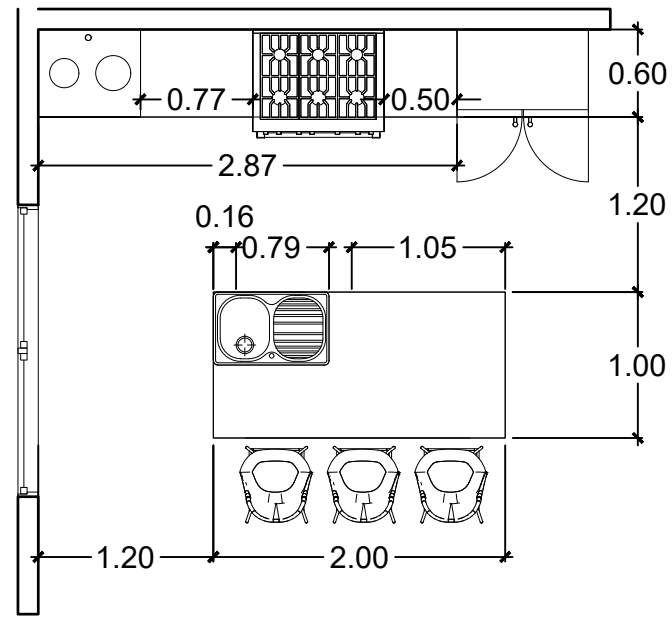
1 COCINA ACOTADA ESCALA: 1:50
