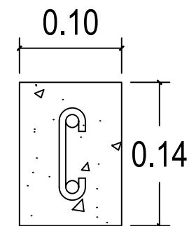
COLUMNA C 2 Ø3/8" + est. Ø1/4" @ 0.20
