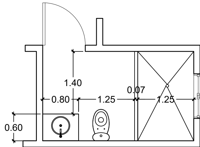
1 S.S. DORMITORIO MASTER ACOTADA ESCALA: 1:50
