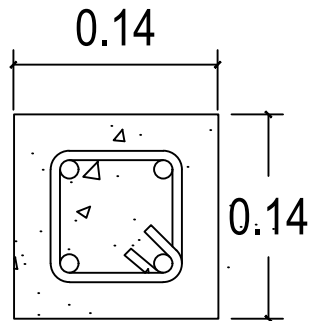
COLUMNA B 4 Ø3/8" + est. Ø1/4" @ 0.15
